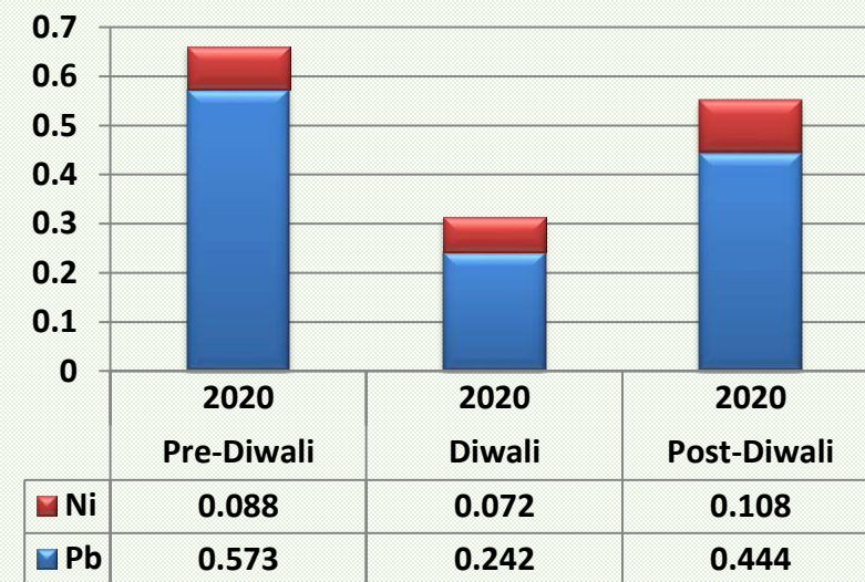
Talkatora
