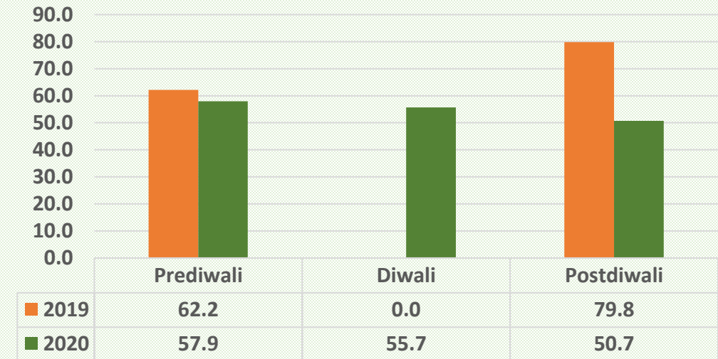
Subros (NO 2 )
