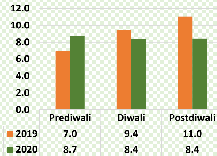
Aliganj
