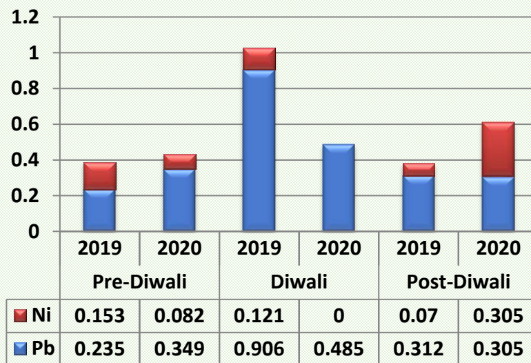
Aliganj
